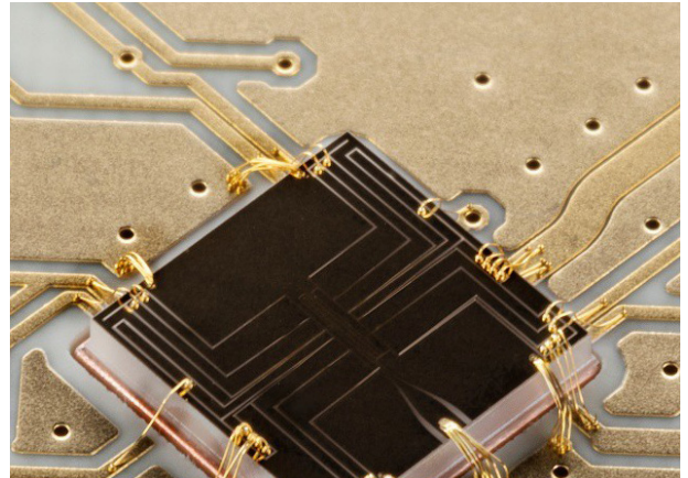
Kontaktierte Oberflächen-Ionenfalle
